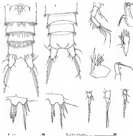
FIG. 1. — Ceuthonectes gallicus . a : abdomen ♀, vue ventrale ; b : abdomen ♀, vue dorsale ; c : A_2 ♀ ; d : mandibule ♀ ; e : maxillule ♀ ; f : maxille ♀ ; g : maxillipède ♀ ; h : P_2 ♂ ; i : P_3 ♂ ; j : endopodite P_2 ♂ ; k : endopodite P_3 ♂ ; l : endopodite P_4 ♂. (Échelle micrométrique.)
